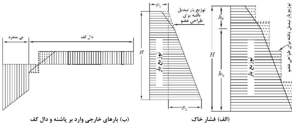
شکل ۴-۲۴- روش تبدیل توزیع بار
