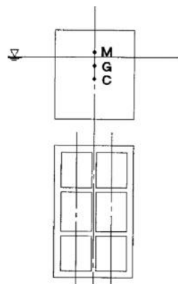
شکل ۴-۳- پایداری صندوقه
