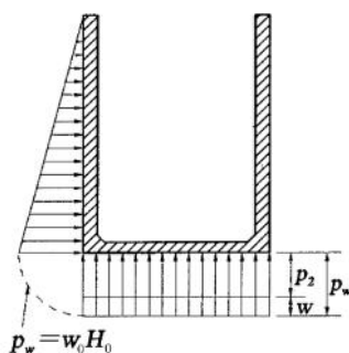
شکل ۴-۱۱- نیروی خارجی وارد بر دال کف
