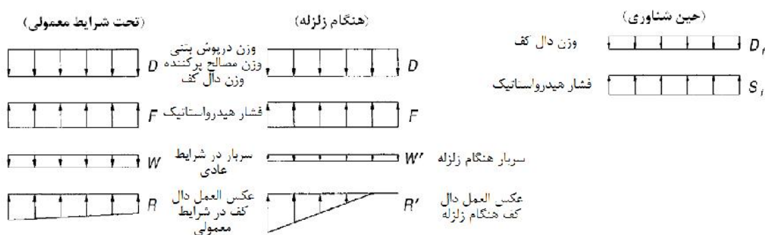
شکل ۴-۹- بارهای طراحی دال‌های کف (دیوار ساحلی)
