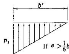
شکل ۴-۱۵- عکس‌العمل کف
