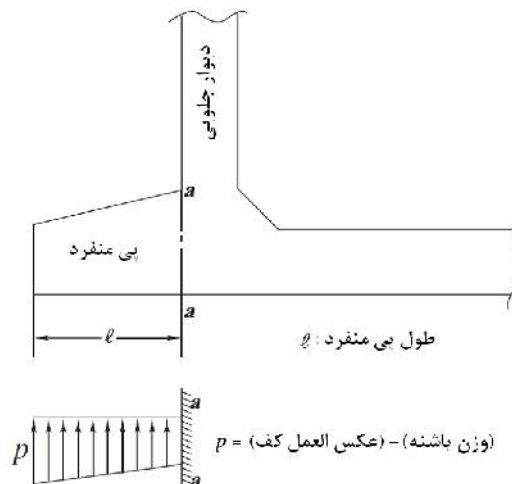
شکل ۴-۲۶- طول و بار پاشنه
