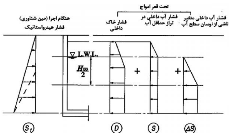
شکل ۴-۶- بارهای طراحی برای دیوار کناری (موج شکن)
